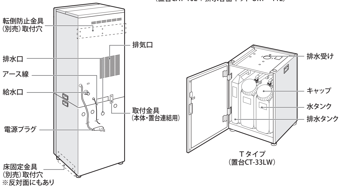
P Bタイプ (置台CAT-10L + 排水容器キット OKT-11L)
