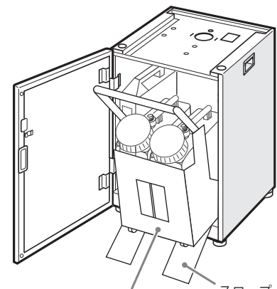
水タンク台車 スロープ
