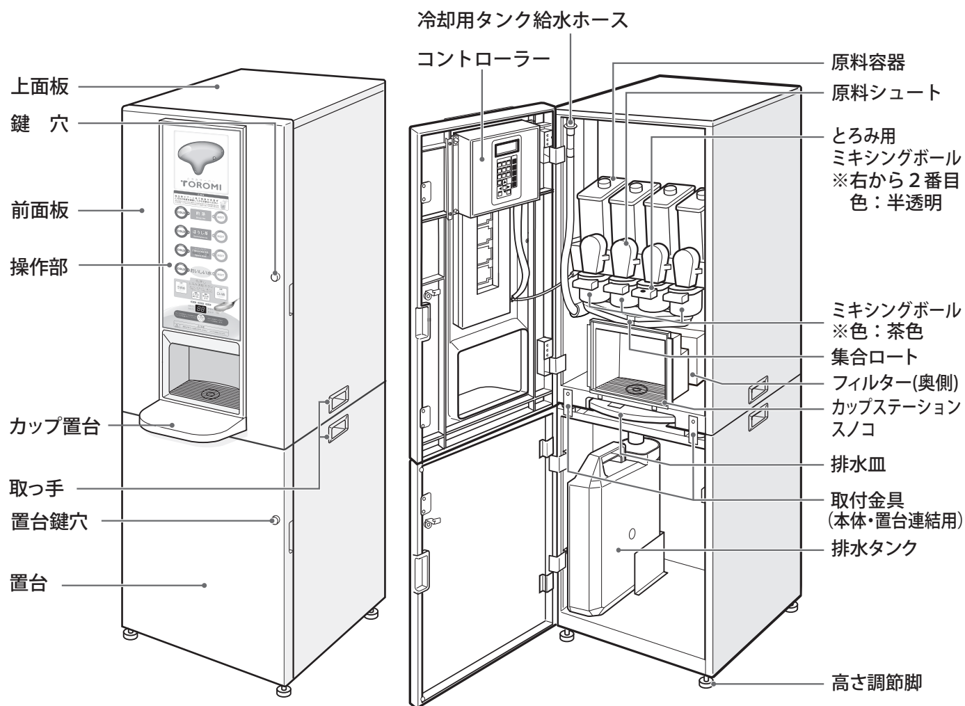
P Bタイプ (置台CAT-10L + 排水容器キット OKT-11L)
